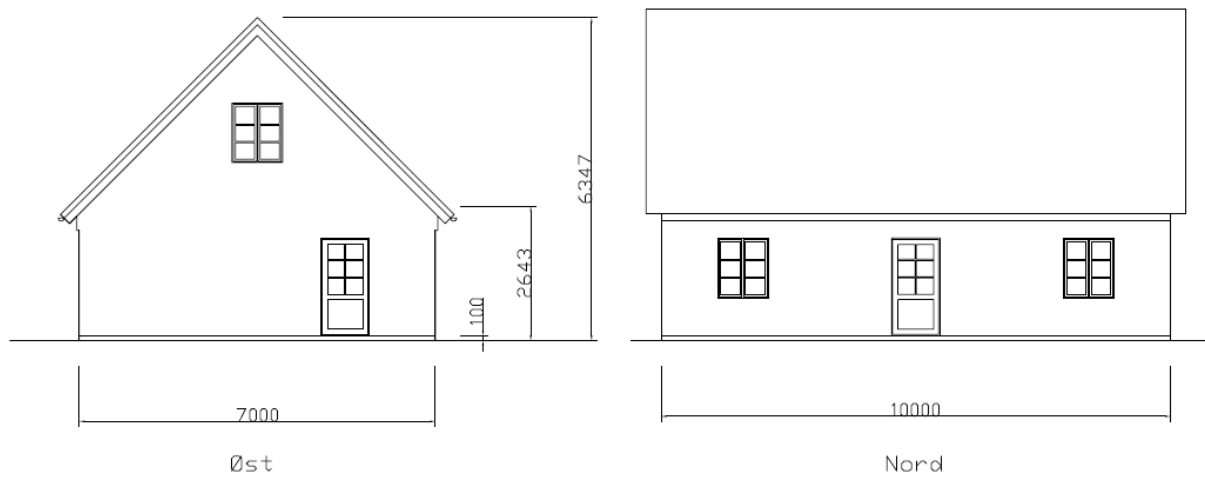
Figur 5. Facade tegning, øst, nord
