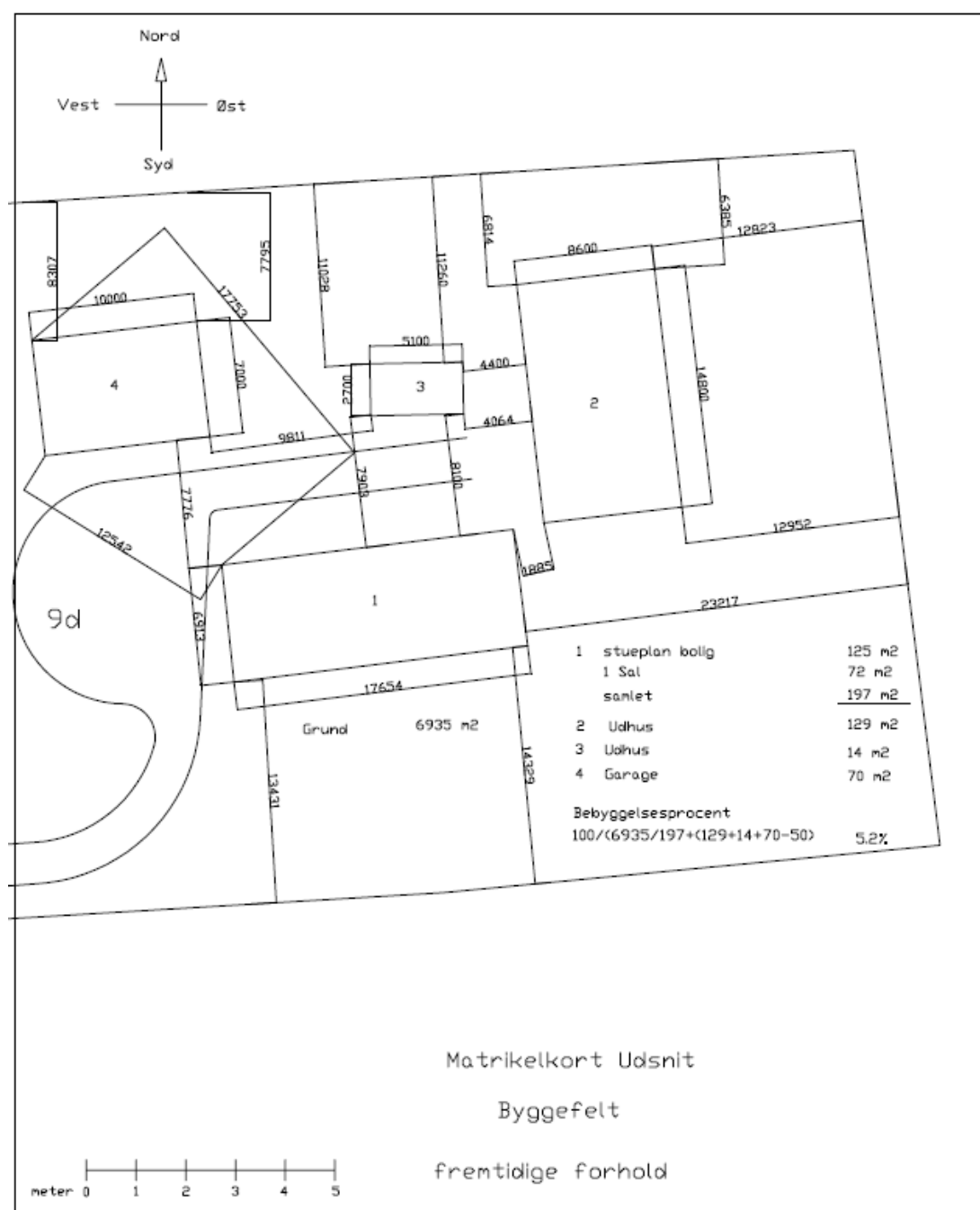
Figur 2. Situationsplan udsnit
