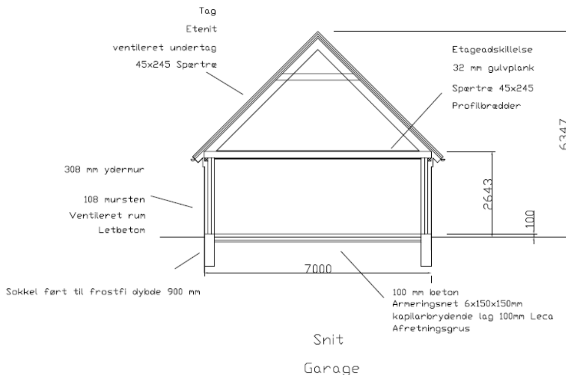
Figur 7. Snit tegning
