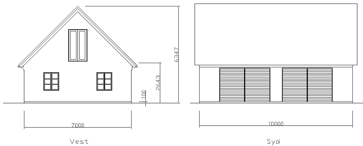
Figur 6. Facade tegning, vest, syd
